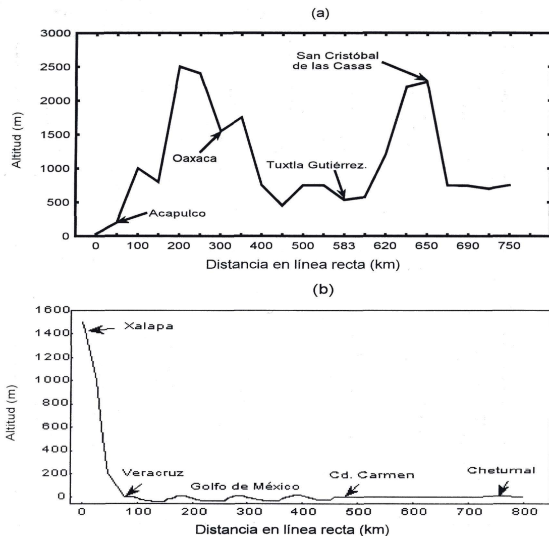
Figura 2. Corte de los transectos a) sur (alrededor del paralelo 17° N, que incluye a las ciudades de Acapulco, Oaxaca, Tuxtla Gutiérrez y San Cristóbal de las Casas) y b) norte (ligeramente al norte del paralelo 19° N, que incluye a las ciudades de Xalapa, Veracruz, Ciudad del Carmen y Chetumal).
