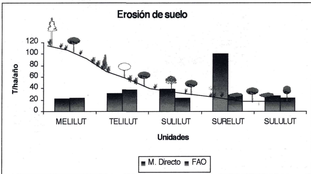
Figura 3. Tasas de erosión de suelo estimadas para cada Unidad Geomorfológica, en comparación con las tasas reales de erosión para 1999. Se incluye un perfil esquematizado mostrando la ubicación de las unidades geomorfológicas con respecto a la pendiente de la microcuenca.
